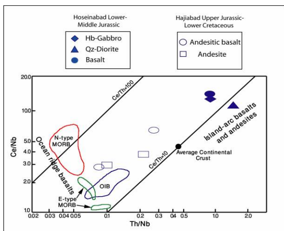
شکل ۱۴- نمودار نسبت Ce/Nb در مقابل نسبت Th/Nb (Saunders and Tarney, 1991) برای تقسیم‌بندی محیط تکتونیکی نمونه‌های ژوراسیک زیرین - میانی حسین‌آباد و ژوراسیک بالایی - کرتاسه زیرین حاجی‌آباد. این نمودار اطلاعات کامل‌تری درباره منشأ و خاستگاه ژئوشیمیایی محیط‌های تکتونیکی مختلف ارائه می‌کند. در این نمودار نمونه‌های حسین‌آباد در محدوده بازالت‌های جزایر قوسی (IAT) و نمونه‌های حاجی‌آباد در محدوده‌های بین بازالت‌های جزایر قوسی (IAT) و مورب غنی شده (E-MORB) تصویر می‌شوند.
