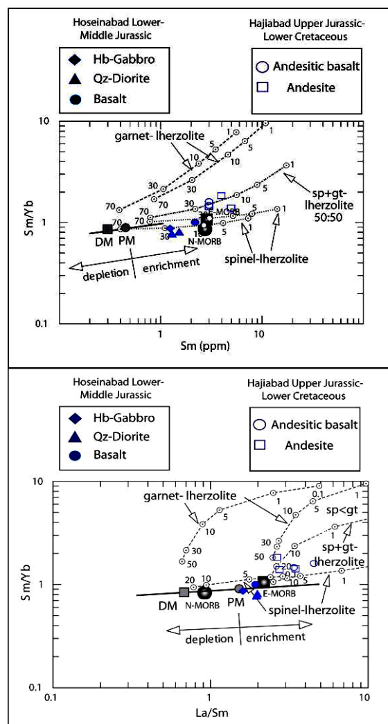
شکل ۱۸- نمودارهای نسبت Sm/Yb در مقابل Sm و نسبت Sm/Yb در برابر نسبت La/Sm برای تعیین درجات ذوب‌بخشی منشأهای گوشته‌ای متفاوت (Aldanmaz et al., 2000) در نمونه‌های ژوراسیک زیرین - میانی حسین‌آباد و ژوراسیک بالایی - کرتاسه زیرین حاجی‌آباد. روند گوشته‌ای (خط ضخیم) توسط ترکیب گوشته تهی شده (DM) (McKenzie and O'Nions, 1991) و گوشته اولیه (PM) (McDonough and Sun, 1995) مشخص می‌شود. منحنی‌های ذوب بخشی برای منشأ گوشته‌ای اسپینل لرزولیت و گارنت لرزولیت با ترکیبات گوشته تهی شده و گوشته اولیه از Aldanmaz و همکاران (۲۰۰۰). ترکیب E-MORB و N-MORB از McDonough و Sun (۱۹۸۹) است. سنگ‌های ژوراسیک زیرین - میانی حسین‌آباد از ذوب بخشی ۱۰ تا ۳۰ درصد یک منشأ گوشته‌ای اسپینل لرزولیت با ترکیب گوشته اولیه (PM) و سنگ‌های ژوراسیک بالایی - کرتاسه زیرین حاجی‌آباد از ذوب بخشی ۱۰ تا ۳۰ درصد یک منشأ گوشته‌ای اسپینل-گارنت لرزولیت با ترکیب مورب غنی شده (E-MORB) حاصل شده‌اند.
