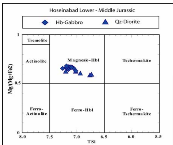
شکل ۱۱- نمودار Mg/(Mg+Fe^{+2}) در مقابل سیلیس تتراهدردی (Leake et al. , 1997). آمفیبول‌ها در نمونه‌های هورنبلند گابرو و کوارتز دیوریت ژوراسیک زیرین - میانی حسین‌آباد دارای ترکیب منیزیهورنبلند هستند.
