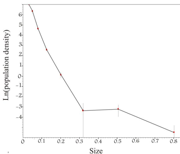
شکل ۱۰- نمودار لگاریتمی چگالی تجمعی در برابر اندازه بلورها برای منطقه قره‌بلاغ
