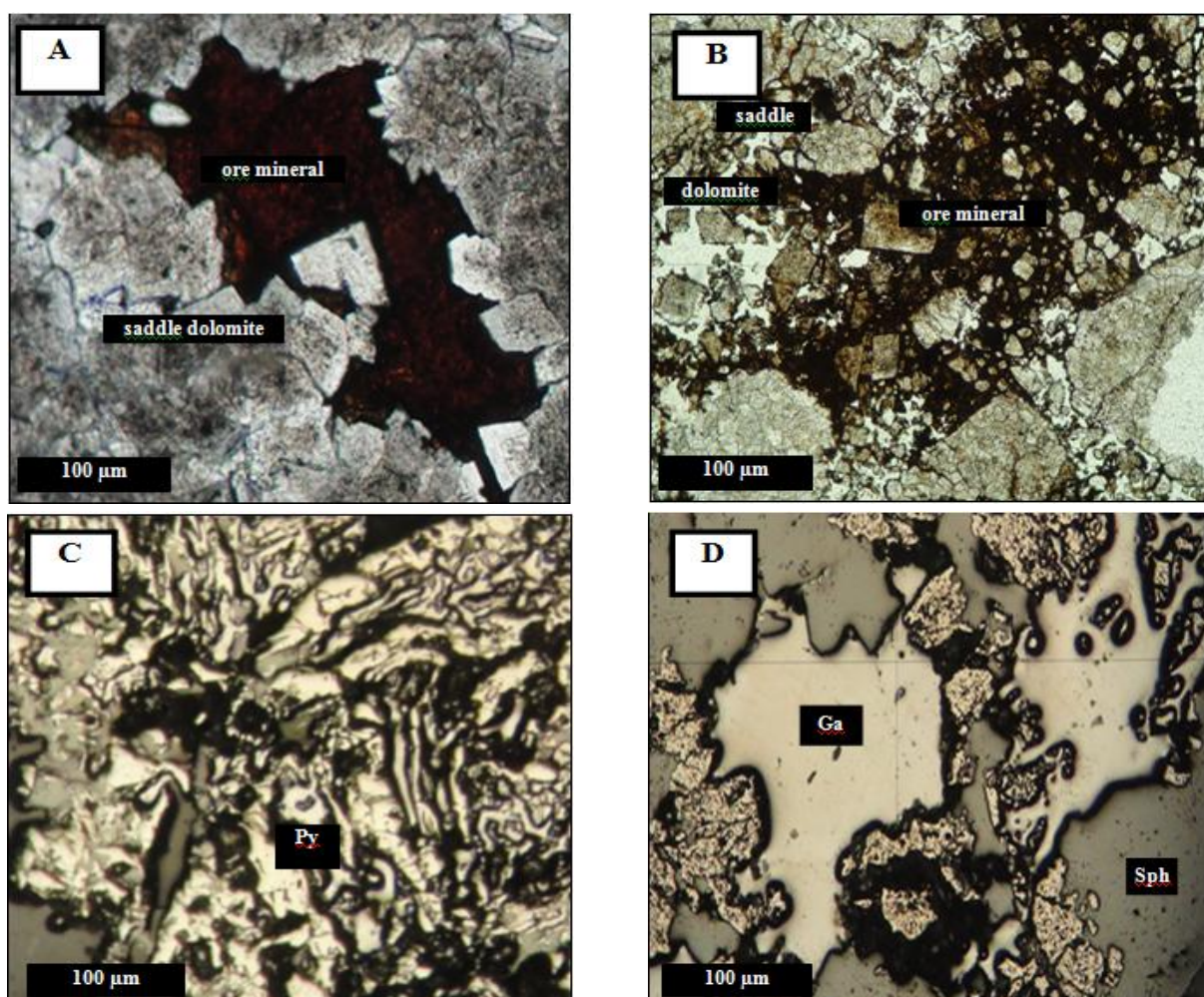
شکل ۳- A و B) رخدادهای معدنی به صورت شکافه پُر کن در دولومیت‌های زین‌اسبی؛ C) پیریت در کوه سورمه، پیش در آمد اسفالریت و گالن است؛ D) بافت هم‌رشدی بین اسفالریت و گالن در کوه سورمه (Ga=گالن، Sph=اسفالریت، Py=پیریت) (تمامی عکس‌ها در نور پلاریزه گرفته شده است).
