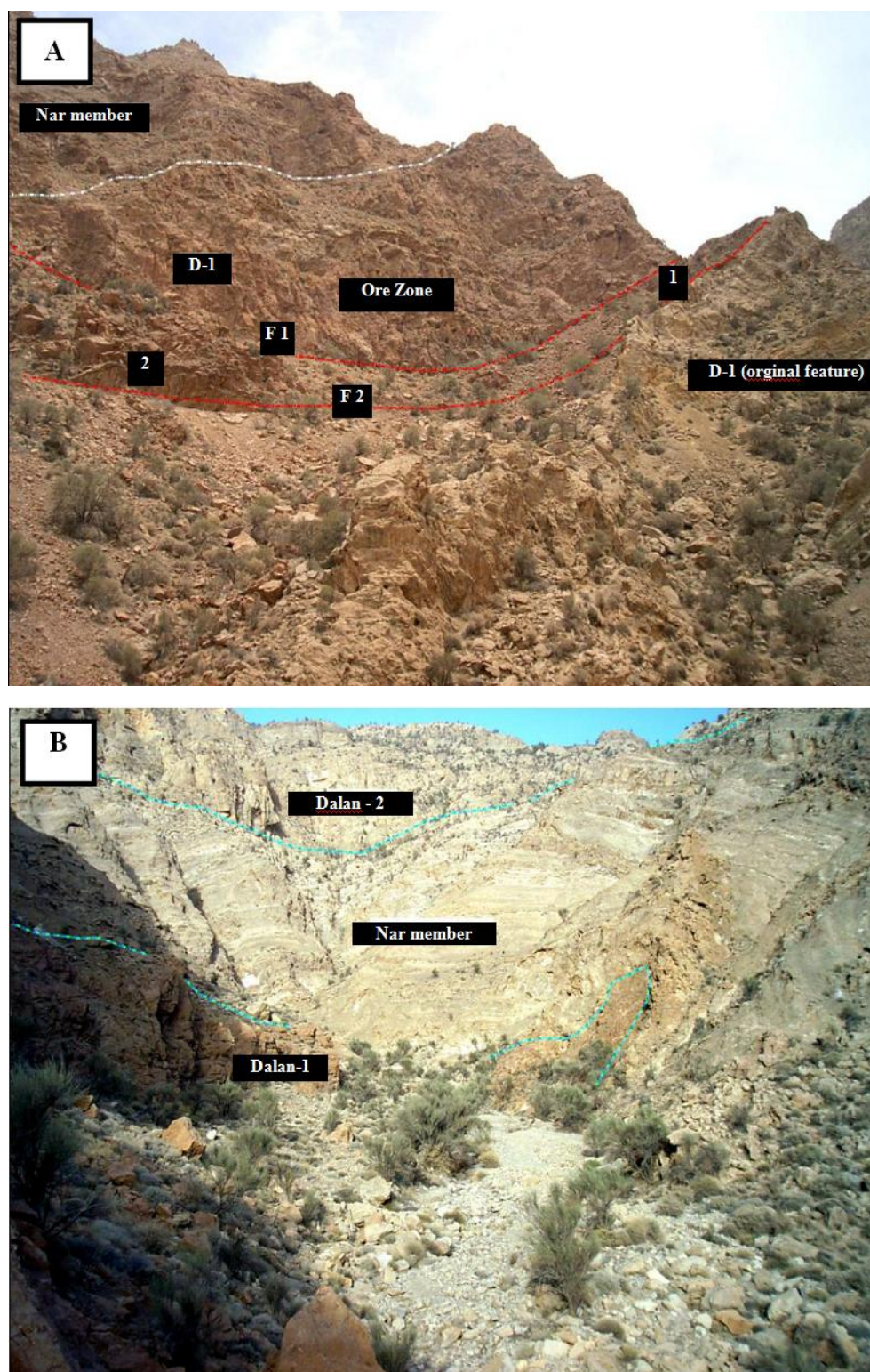
شکل ۲- A) ساختار پهنه گسلیده اصلی (1) و وضعیت پهنه مینرالیزه در فرادیواره شمال شرقی (گسل‌های منطقه = F1 و F2، دالان زیرین = D-1؛ B) نمایی از سازند دالان یک و دو که توسط عضو تبخیری نار از هم جدا شده‌اند.
