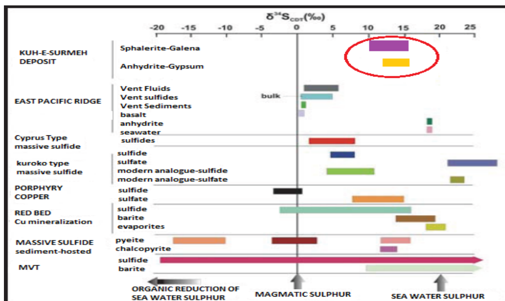
شکل ۷- تغییرات \delta^{34}\text{S} در محیط‌های مختلف زمین‌شناسی (Rollinson, 1995) و جایگاه محدوده تغییرات \delta^{34}\text{S} کانی‌های سولفیدی و سولفاتی کانسار کوه سورمه
