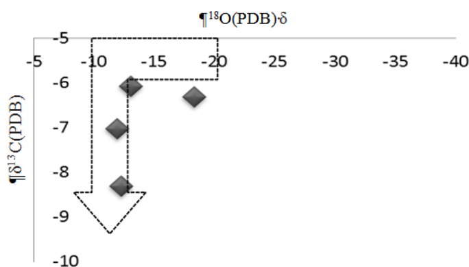
شکل ۶- تغییرات مقادیر \delta^{18}\text{O}_{\text{PDB}} در مقابل \delta^{13}\text{C}_{\text{PDB}} در کانسار کوه سورمه
