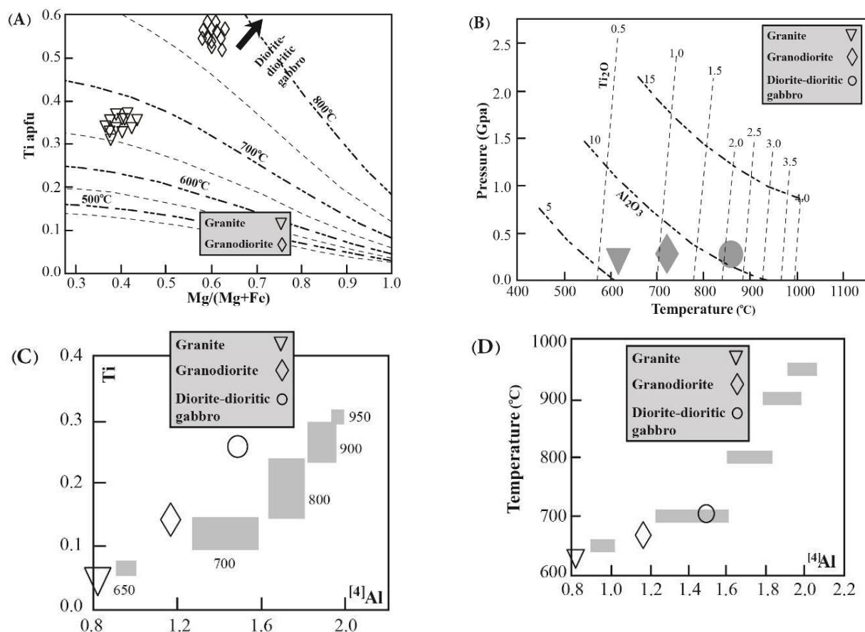
شکل ۷- نمودارهای حرارت‌سنج و فشارسنج توصیفی بر اساس ترکیب شیمیایی بیوتیت و آمفیبول: (A) مقدار Ti در فرمول شیمیایی بیوتیت در مقابل مقدار XFe (Henry and Guidotti, 2002) (B) تعیین مقدار فشار و حرارت بر اساس منحنی‌های هم‌ترکیبی TiO 2 و Al 2 O 3 بلورهای آمفیبول (Ernst and Liu, 1998) (C) و (D) تعیین دمای تشکیل آمفیبول‌ها بر اساس مقدار Ti و [Al] (Ernst and Liu, 1998).
