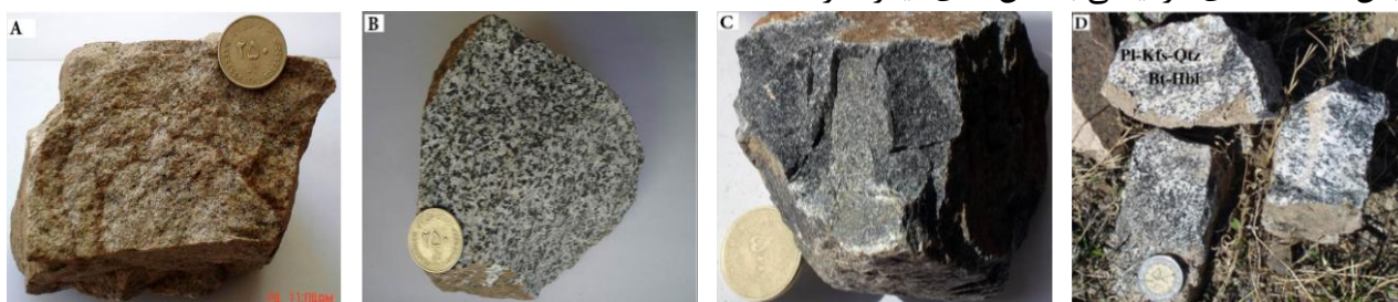
شکل ۲- تصاویری از نمونه‌های دستی انواع سنگ‌های موجود در باتولیت تخت: (A) آلکالی‌فلدسپارگرانیت؛ (B) گرانودیوریت؛ (C) گابروی دیوریتی؛ (D) تبلور تفریقی و جدایش بلورهای مختلف
