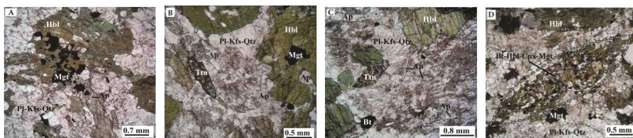
شکل ۳- تصاویر میکروسکوپی انتخابی از رخنمون‌های مختلف سنگی: (A) تصویر میکروسکوپی از مونزوگرانیت؛ (B) تصویر میکروسکوپی از سنگ‌های گرانودیوریت. بلورهای آپاتیت سوزنی و منشوری همراه با تیتانیت و مگنتیت مشاهده می‌شود؛ (C) تصویر میکروسکوپی از گرانودیوریت همراه با بلورهای سوزنی آپاتیت و بلورهای تیتانیت؛ (D) آنکلاو میکروگرانولار مافیک با تجمعی از بلورهای بیوتیت، هورنبلند، کلینوپیروکسن و مگنتیت. اختصارات کانی‌ها از Kretz (۱۹۸۳) است.
