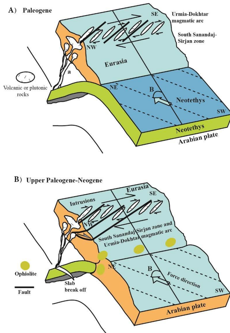
شکل ۸- مدل تکتونیکی تشکیل باتولیت تخت در بخش جنوبی کمربند ماگمایی ارومیه-دختر. فروورانش مایل نه تنها باعث ذوب بخشی بلکه باعث ایجاد فضای لازم برای تزریق این باتولیت شده است.
