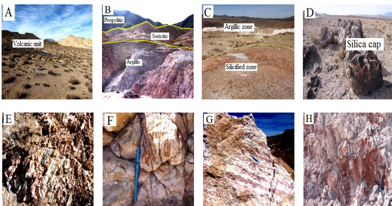
شکل ۳- تصاویر صحرایی. (A) واحدهای ولکانیکی؛ (B) رخنمونی از واحدهای دگرسان منطقه؛ (C) تفکیک بقایای پهنه سیلیسیک با آرژیلیک (این تفکیک فرضی است و گاهی جدایش، در سطح قطعاً میسر نیست)؛ (D) کلاهدک سیلیسی؛ (E) نمای لایه‌ای از پهنه سریستیک؛ (F) حلقه‌های رنگین در پهنه سریستیک؛ (G) دگرسانی کائولن با حفظ بافت اولیه سنگ میزبان دگرسانی (ایگنیمبریت)؛ (H) پهنه آرژیلیک آغشته به اکسید آهن.
