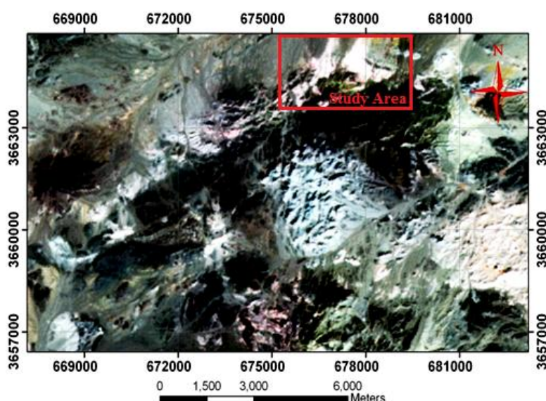
شکل ۲- تصویر پردازش شده اطلاعات ماهواره‌ای (RGB 468) منطقه شمال نایین با استفاده از داده‌های استر. کانی‌های دارای بنیان OH به رنگ صورتی متمایل به سفید و کلریت و اپیدوت به رنگ سبز.
