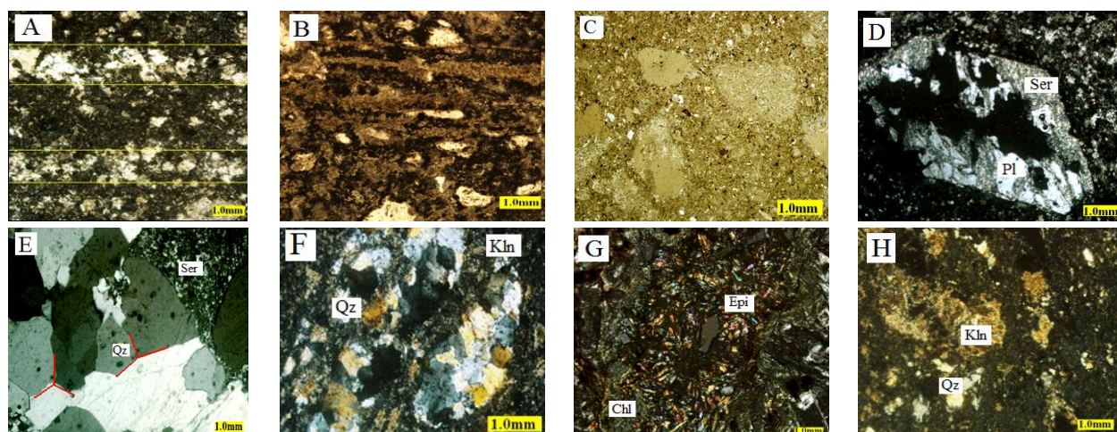
شکل ۴- تصاویر میکروسکوپی. (A) واحد آذر آواری ایگنمبریتی (XPL)؛ (B) بافت اوتاکسیتیک در ایگنمبریت (PPL)؛ (C) بافت شبحی از بافت پیروکلاستیک توف اولیه که دچار دگرسانی فراگیر شده است (PPL)؛ (D) تبدیل پلاژیوکلاز به سیریسیت (XPL)؛ (E) کوارتز پلی‌کریستالین با بافت پلی‌گوناال (موزاییکی) (XPL)؛ (F) کوارتزهای بی‌شکل به صورت پرکننده حفرات در یک زمینه کائولینیتی (XPL)؛ (G) کلریتی و اپیدوتی شدن در آندزیت بازالت (XPL)؛ (H) همیافتی کائولینیت (جزو اصلی پهنه آرژیلیک) با کوارتز (XPL). علایم اختصاری اقتباس از Whitney و Evans (۲۰۱۰).
