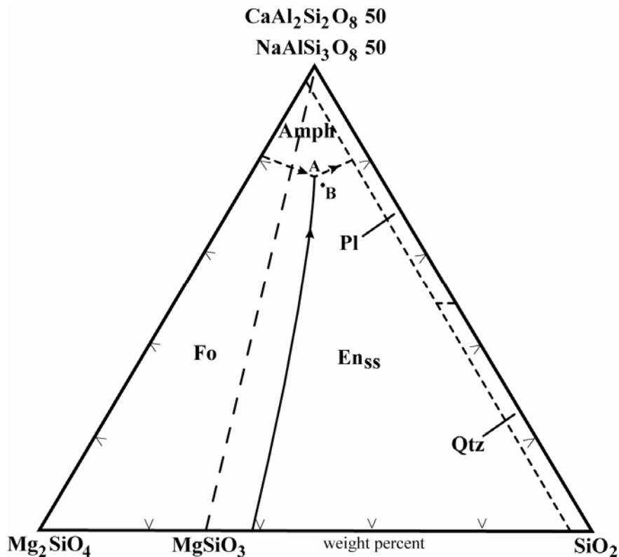
شکل ۶- نمودار لیکیدوس متعادل سیستم فورستریت ( Mg_2SiO_4 )-پلاژیوکلاز ( CaAl_2Si_2O_8 50 wt% - NaAlSi_3O_8 50 wt%) -سیلیکا ( SiO_2 ) - آب ( H_2O ) در ۱۵ کیلو بار. مرزهای لیکیدوس تحت شرایط بخار آب در نقطه A در دماهای 1000 \pm 20 ، فورستریت+محلول جامد+آمفیبول+مایع+بخار است. خطوط خط‌چین مرزهای لیکیدوس فورستریت-محلول جامد انستاتیت و محلول جامد انستاتیت-آمفیبول هستند و نقطه B تخمین نقطه است که KAlSi_3O_8 ۱۰ درصد وزنی در سیستم فورستریت-پلاژیوکلاز-آرتوکلاز-سیلیکا-آب در ۱۵ کیلو بار است ( Qtz = کوارتز، Pl = پلاژیوکلاز، Amph = آمفیبول، Fo = فورستریت، En_{ss} = محلول جامد فورستریت).
