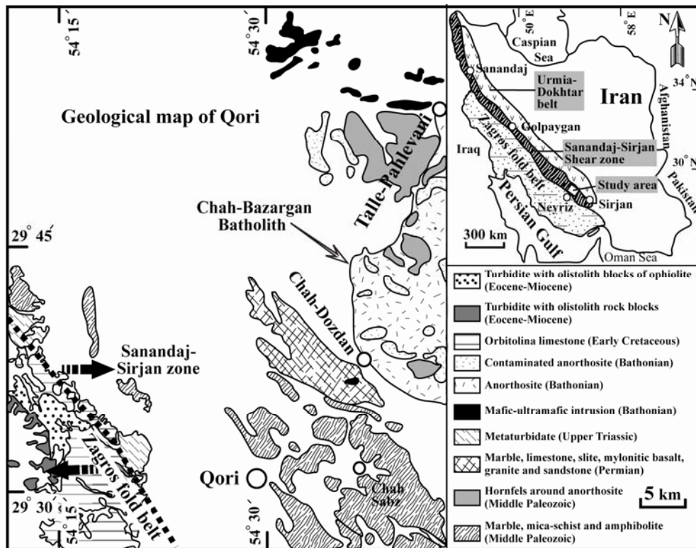
شکل ۱- نقشه زمین‌شناسی ساده شده محدود شمال شرق نیریز (با تغییرات، از سبزی و همکاران، ۱۳۷۲).
