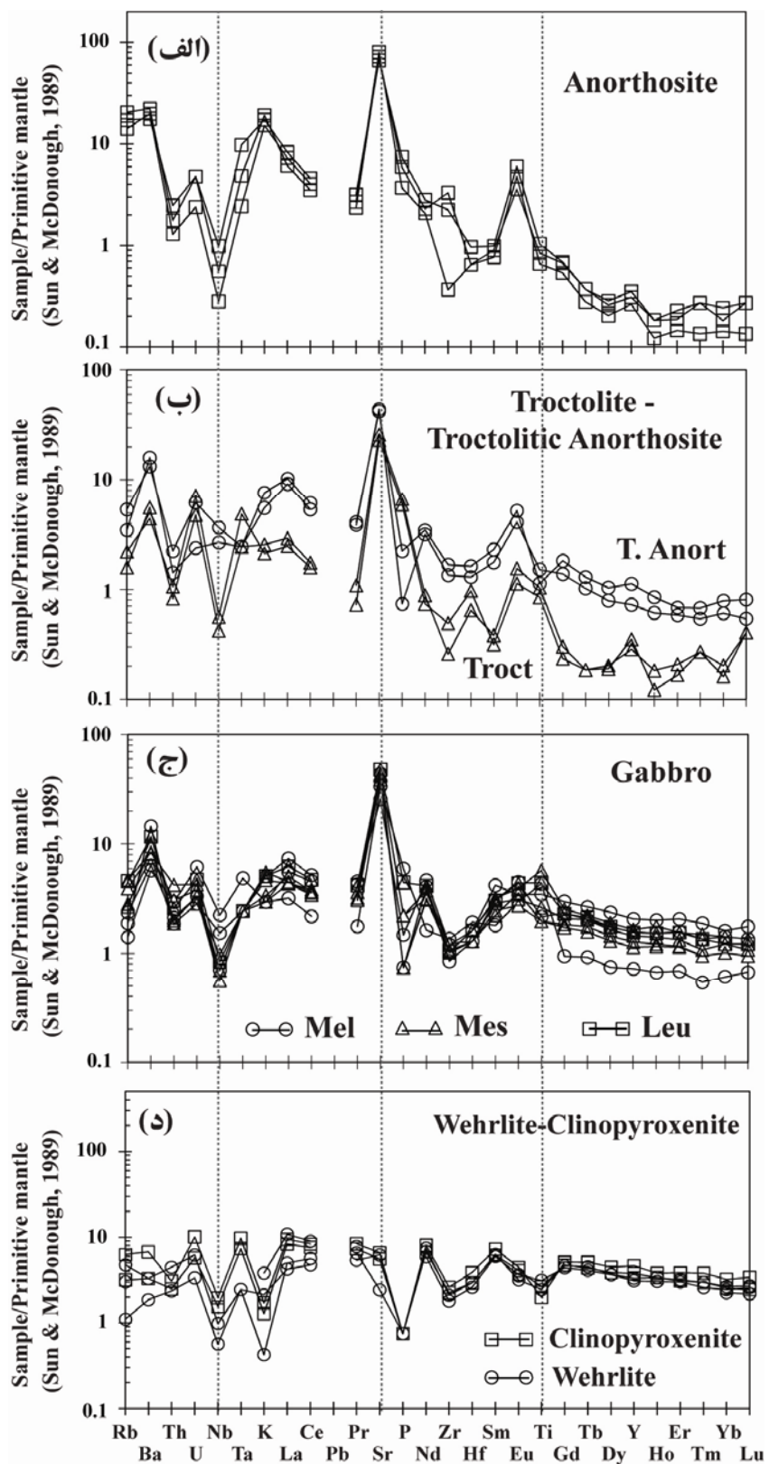
شکل ۴- نمودارهای عنکبوتی چند عنصری برای انواع سنگ‌های رخنمون یافته در نفوذی‌های مافیک-اولترامافیک تله‌پهلوانی. نورمالیز بر اساس گوشته اولیه از Sun and McDonough (1989). مخفف‌ها: Leu=لوکوگابرو؛ Mel=ملاگابرو؛ Mes=مزوگابرو؛ Troct=تروکتولیت؛ T.Anort=آنورتوزیت تروکتولیتی.
