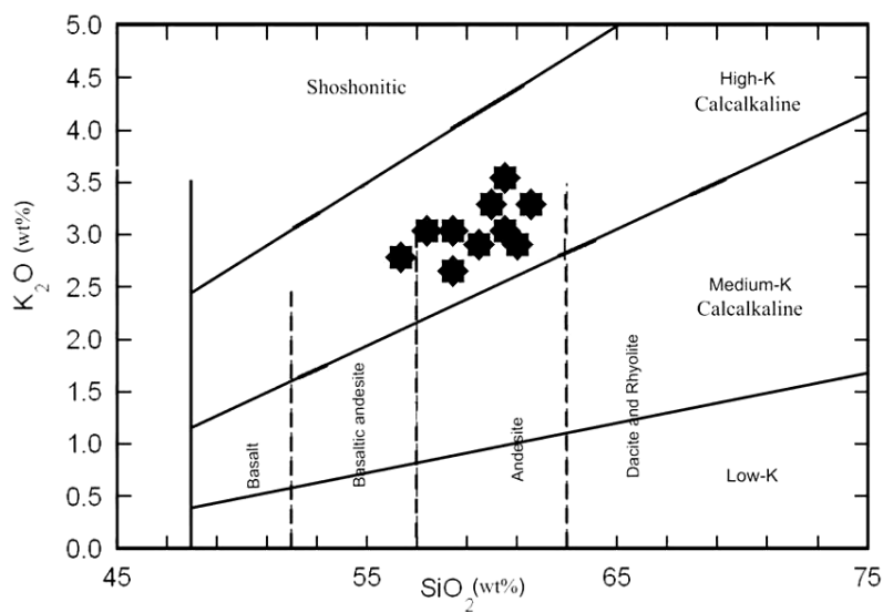
شکل ۶ - نمودار K_2O در مقابل SiO_2 (LeMaitre et al. , 1989) و موقعیت سنگ‌های آتشفشانی منطقه حسین‌آباد
