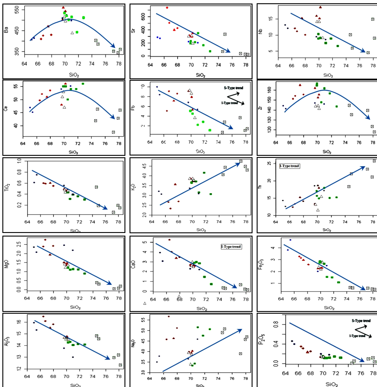
شکل ۵- جایگاه و روند تغییرات نمونه‌های توده‌های گرانیتوئیدی یزد بر روی نمودار اکسیدهای عناصر اصلی و کمیاب در مقابل SiO 2
