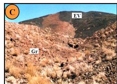
شکل ۲- ارتباط صحرایی توده‌های نفوذی یزد با سنگ‌های منطقه: (A) کنتاکت توده گرانیتوئیدی (Gr) با سازند کهر (KF)، (B) کنتاکت توده گرانیتوئیدی (Gr) با سازند تفت (TF) و اسکارن‌زایی (S) و (C) نفوذ زبانه‌هایی از توده در سنگ‌های آتشفشانی ائوسن (EV)
