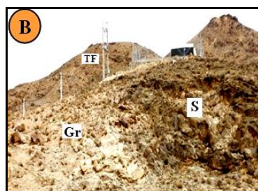
شکل ۲- ارتباط صحرایی توده‌های نفوذی یزد با سنگ‌های منطقه: (A) کنتاکت توده گرانیتوئیدی (Gr) با سازند کهر (KF)، (B) کنتاکت توده گرانیتوئیدی (Gr) با سازند تفت (TF) و اسکارن‌زایی (S) و (C) نفوذ زبانه‌هایی از توده در سنگ‌های آتشفشانی ائوسن (EV)
