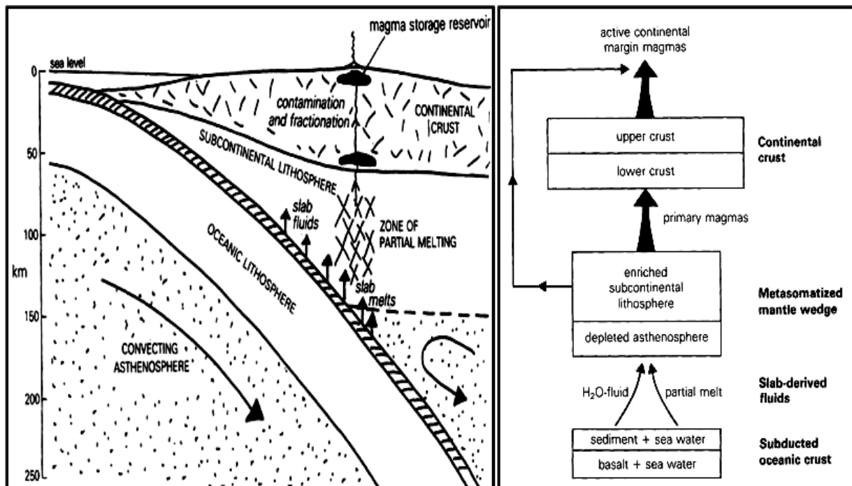
شکل ۸- مدل ژئودینامیکی پیشنهادی Wilson (۲۰۰۷) و فرآیندهای مؤثر در تشکیل ماگمای حاشیه فعال قاره‌ای
