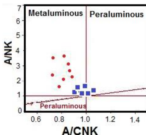
شکل ۷- نمودار A/NK در مقابل A/CNK (Maniar and Piccoli, 1989). قرارگیری نمونه‌ها در محدوده متآلومین. علایم مشابه شکل ۳ است.
