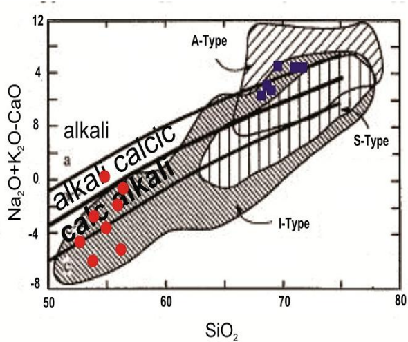
شکل ۶- نمودار SiO_2 در برابر Na_2O+K_2O-CaO (Frost et al., 2001). قرار گیری نمونه‌ها در محدوده گرانیت‌های نوع I کالک‌آلکان و آلکالی کلسیک. علایم مشابه شکل ۳ است.
