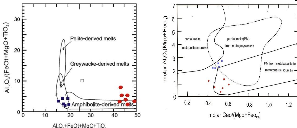
شکل ۱۲- قرارگیری نمونه‌های توده نفوذی در محدوده ذوب گریوک‌ها و قرارگیری نمونه‌های دایک‌ها در محدوده ذوب آمفیبولیت‌ها (Patino Douce, 1999). علایم مشابه شکل ۳ است.
