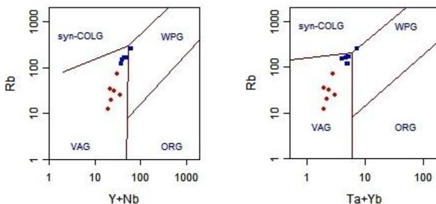
شکل ۱۰- نمودارهای Rb-(Y+Nb) و Rb-(Ta+Yb) برای تفکیک انواع گرانیته‌های پشته‌های میان اقیانوسی (ORG)، گرانیته‌های کمان آتشفشانی (VAG)، گرانیته‌های درون صفحه‌ای (WPG) و گرانیته‌های همزمان با برخورد (syn-COLG) (Pearce et al. , 1984). علایم مشابه شکل ۳ است.
