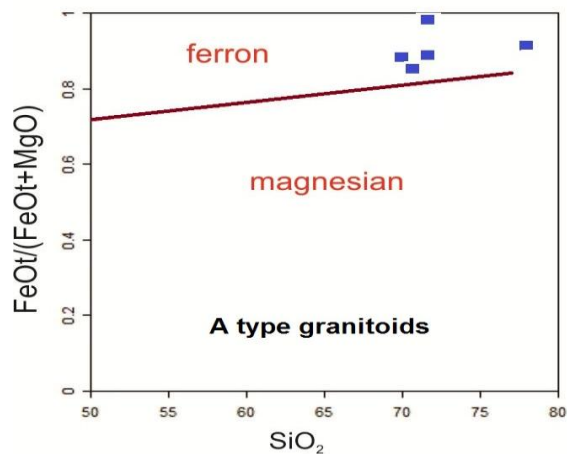
شکل ۵- موقعیت نمونه‌های گرانیتی نصرند بر روی نمودار تفکیک گرانیت‌های Mg دار از انواع Fe دار (Frost et al., 2001).
