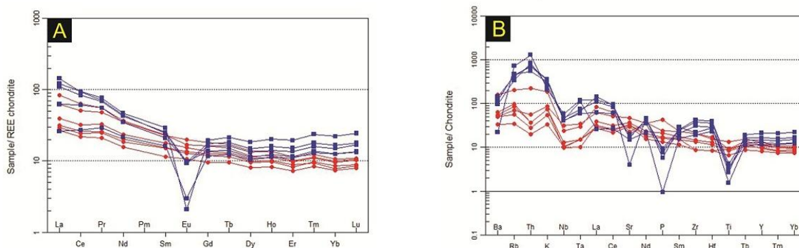
شکل ۹- نمودار بهنجار شده عناصر نادر خاکی گرانیت‌ها و دایک‌ها نسبت به عناصر کمیاب در کندریت‌ها (Nakamura, 1974)؛ (B) نمودار بهنجار شده عناصر کمیاب نمونه‌های گرانیتی و دلریتی نسبت به کندریت (Thompson, 1982). علایم مشابه شکل ۳ است.
