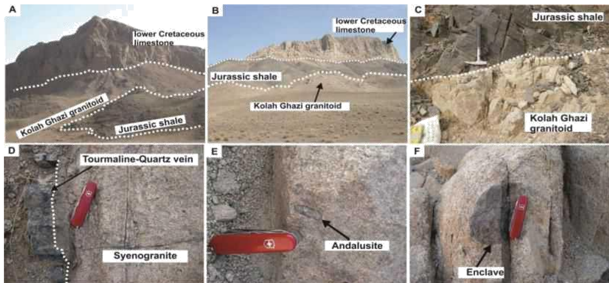
شکل ۲- تصاویرهای صحرایی از توده گرانیتوئیدی کلاه‌قازی (جنوب‌باختری اصفهان). A، B) جایگاه و رخمون توده گرانیتوئیدی کلاه‌قازی در منطقه لاگور که در میان شیل‌های ژوراسیک تزریق و توسط آهک کرتاسه پیشین پوشانده شده است در منطقه لاگور بزرگ؛ C) مرز بین توده کلاه‌قازی و شیل‌های دگرگون‌شده (اسلیت)؛ D) رگه کوارتز-تورمالینی در سینوگرانیت‌های کلاه‌قازی؛ E) درشت بلورهای آندالوزیت در گرانیتوئید کلاه‌قازی؛ F) انکلاو غنی از بیوتیت در گرانیتوئید کلاه‌قازی.
