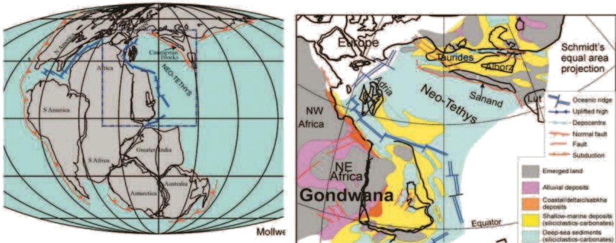
شکل ۸- بازسازی جغرافیای دیرینه کالوین (۱۶۴ میلیون سال پیش) حوضه تتیس بر اساس Berra و Angiolini (۲۰۱۴).
