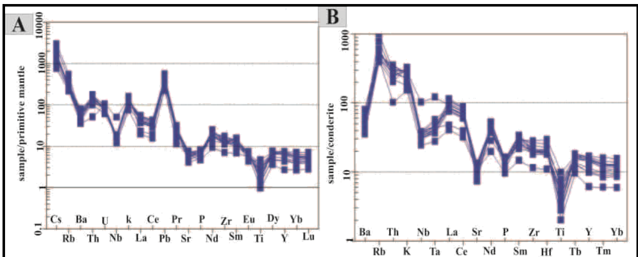
شکل ۵- ترکیب شیمی سنگ کل واحدهای سنگی توده گرانیتوئیدی کلاهقازی در نمودار: (A) الگوی چند عنصری به‌هنگار شده نسبت به ترکیب گوشته اولیه (Sun and McDonough, 1989)؛ (B) الگوی عناصر خاکی نادر به‌هنگار شده نسبت به ترکیب کندریت (Thompson, 1982).
