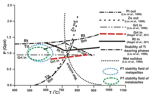
شکل ۷- شبکه سنگ‌زادی گذر از رخساره آمفیبولیت به اکلوزیت و نمودار پایداری فازهای تیتانیم‌دار در ترکیبات مورب (MORB) آبدار (Liu et al., 1996).
