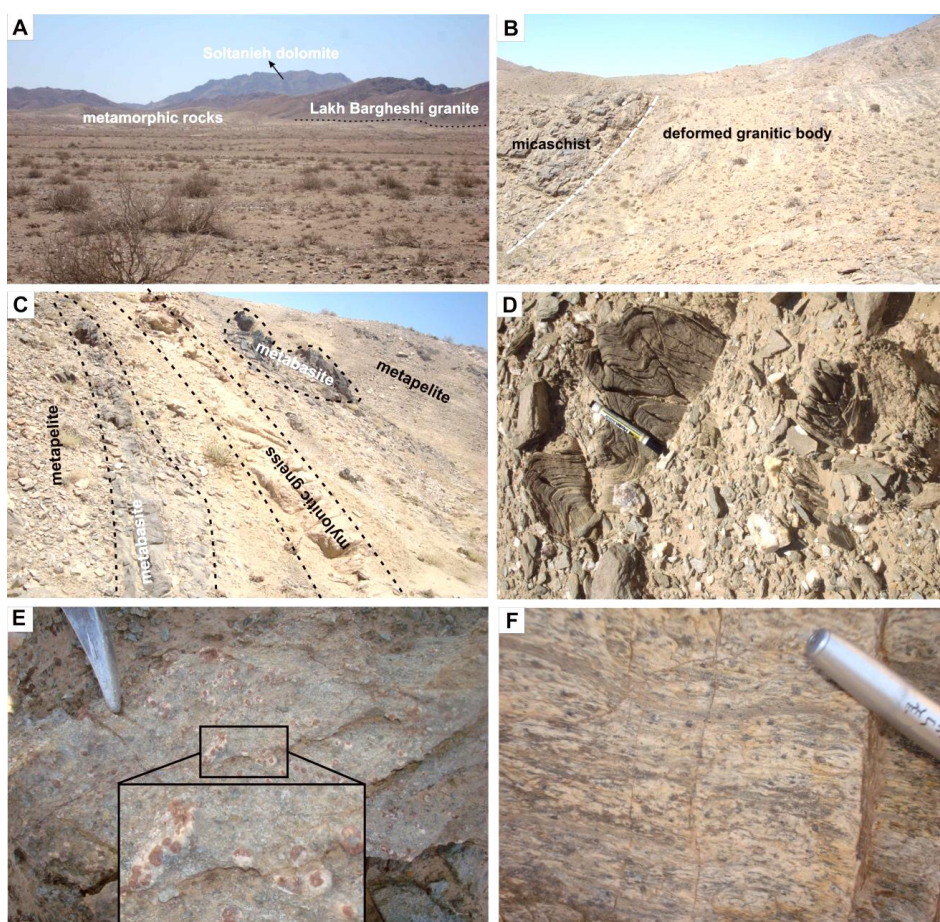
شکل ۲- نمای صحرائی رخنمون پی‌سنگ دگرگونی پرکامبرین ایران مرکزی در منطقه لاخ برقی (جنوب‌باختر بردسکن، خراسان رضوی). (A) دورنمایی از پی‌سنگ دگرگونی پرکامبرین ایران مرکزی در منطقه لاخ برقی. سنگ‌های دگرگونی حالت تپه ماهوری داشته، توده گرانیبی لاخ برقی در آن نفوذ کرده است. گرانیب لاخ برقی و سازند دولومیت سلطانیه، سازنده ارتفاعات منطقه است؛ (B) همبری گسله بین گرانیب لاخ برقی و متاپلیت میزبان؛ (C) تناوب متاپلیت، متابازیت و گنیس میلونیتی در سنگ‌های دگرگونی منطقه؛ (D) دگرشکلی متاپلیت‌ها به صورت چین‌خوردگی؛ (E) هاله فقیرشدگی روشن متشکل از کوارتز و فلدسپار در اطراف پورفیروبلاست‌های گارنت؛ (F) باند گنیس میلونیتی در سنگ میزبان متاپلیتی.
