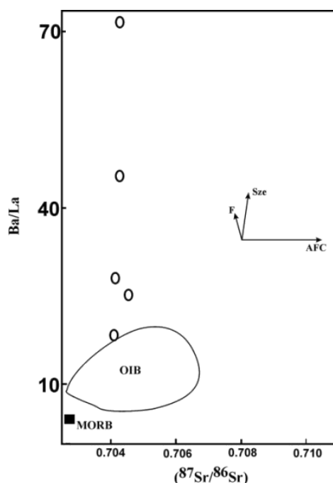
شکل ۸- سنگ‌های آتشفشانی خونیک (جنوب بیرجند، خراسان جنوبی) در نمودار Ba/La در برابر (^{87}Sr/^{86}Sr) (Davidson, 1987) (SZE: پهنه فرورانش، AFC: آغستگی پوسته‌ای، F: تأثیر احتمالی جدایش بلورین).
