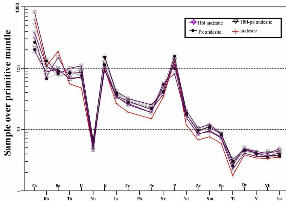
شکل ۷- سنگ‌های آتشفشانی خونیک (جنوب بیرجند، خراسان جنوبی) در نمودار عنکبوتی عناصر فرعی و کمیاب که در برابر ترکیب گوشته اولیه (Sun and McDonough, 1989) به‌نچار شده است.
