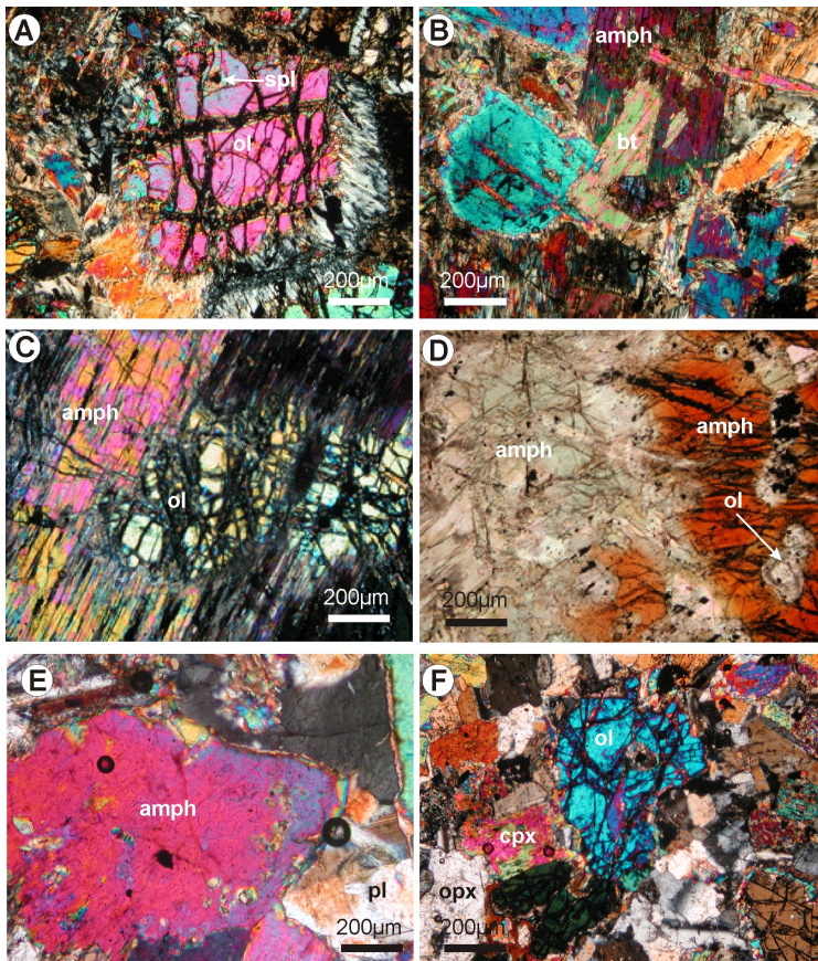
شکل ۳- تصاویرهای میکروسکوپی از الترامافیک‌های ملاطالب (شمال‌باختری الیگودرز، لرستان). A) بلور الیون با میانبار اسپینل درون؛ B) کانی فرعی بیوتیت؛ C) بلورهای بی‌شکل الیون به صورت میانبارهایی درون آمفیبول؛ D) آمفیبول‌های نوع قهوه‌ای و سبز به همراه میانبار الیون (بخش حاشیه‌ای آمفیبول قهوه‌ای با آمفیبول سبز پوشیده شده است)؛ E) رویداد آمفیبول و پلاژیوکلاز در کنار هم؛ F) بلورهای ارتوپروکسن، کلینوپروکسن و آمفیبول که در کنار یکدیگر جای گرفته‌اند (همه تصاویرها در XPL هستند، مگر تصویر D که PPL است)
