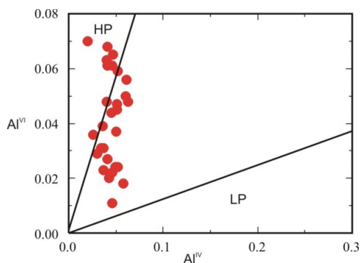
شکل ۱۳- ارزیابی میزان فشار برای الترامافیک‌های ملاطالب (شمال‌باختری الیگودرز، لرستان) برپایه توزیع آلومینیم در جایگاه اکتاهدردی و تتراهدردی ساختار پیروکسن (Aoki and Shiba, 1973)
