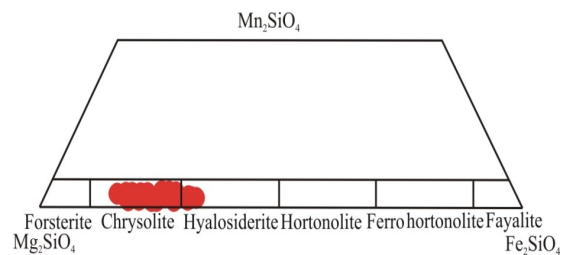
شکل ۷- الیون‌های درون الترامافیک‌های ملاطاب (شمال‌باختری الیگودرز، لرستان) در نمودار رده‌بندی الیون‌ها (Cornelius and Corneli, 1985)
