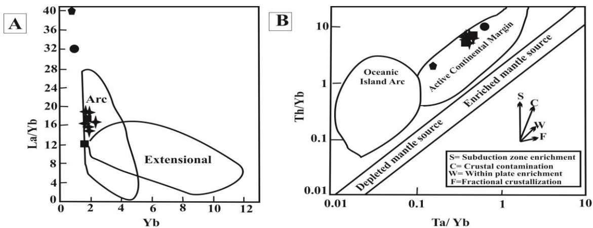
شکل ۱۲- جایگاه سنگ‌های آتشفشانی خاور خوسف در نمودارهای: (A) \text{Yb} در برابر \text{La/Yb} (Pearce, 1983)؛ (B) \text{Ta/Yb} در برابر \text{Th/Yb}
