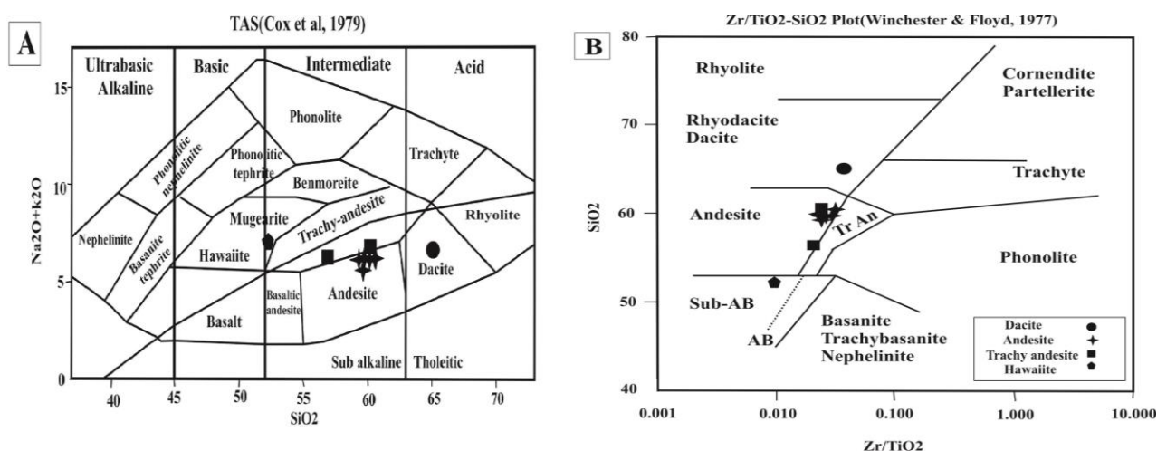
شکل ۸- جایگاه سنگ‌های آتشفشانی خاور خوسف در: (A) نمودار رده‌بندی TAS برپایه SiO_2 در برابر Na_2O+K_2O (Cox et al., 1979); (B) نمودار تغییری رات Zr/TiO_2 در برابر SiO_2 (Winchester and Floyd, 1977)
