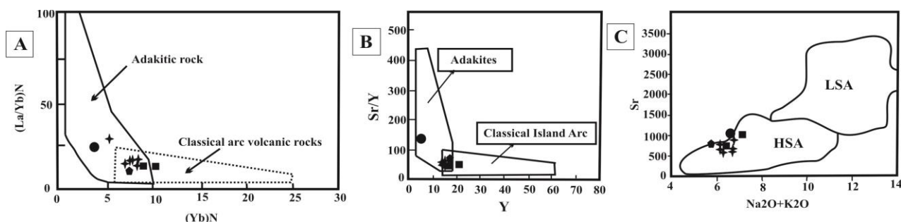
شکل ۱۱- جایگاه سنگ‌های آتشفشانی خاور خوسف در نمودارهای جداکننده سنگ‌های کالک‌آلکان معمولی از آداکیت‌ها: (A) نمودار \text{La}/\text{Yb}_N در برابر \text{Yb}_N (Reich et al., 2003)؛ (B) نمودار Y در برابر Sr/Y (Drummond and Defant, 1990)؛ (C) نمودار \text{Na}_2\text{O}+\text{K}_2\text{O} در برابر Sr (Castillo, 2012)
