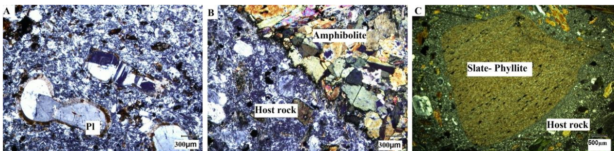
شکل ۵- ویژگی‌های میکروسکوپی داسیت‌های خاور خوسف (جنوب‌باختری بیرجند): (A) بافت پورفیریتیک با خمیره میکروکریستالین و حاشیه قهوه‌ای گردآگرد پلاژیوکلازها و ماکل کارلسباد و پلی‌سینتیک در پلاژیوکلازها و نیز بلورهای سوزنی هورنبلند در داسیت‌ها؛ (B) برونبوم آمفیبولیتی؛ (C) برونبوم متاپلیتی (نور در همه شکل‌ها XPL است)
