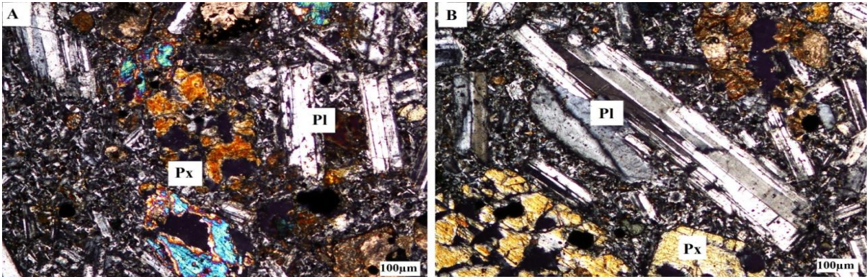
شکل ۷- ویژگی های میکروسکوپی میکرودیوریت منطقه خاور خوسف (در XPL): (A) بافت پورفیریتیک با زمینه دانه ریز؛ (B) فنوکریست های پلاژیوکلاز و کلینوپیروکسن در زمینه دانه ریز ساخته شده از میکرولیت های پلاژیوکلاز
