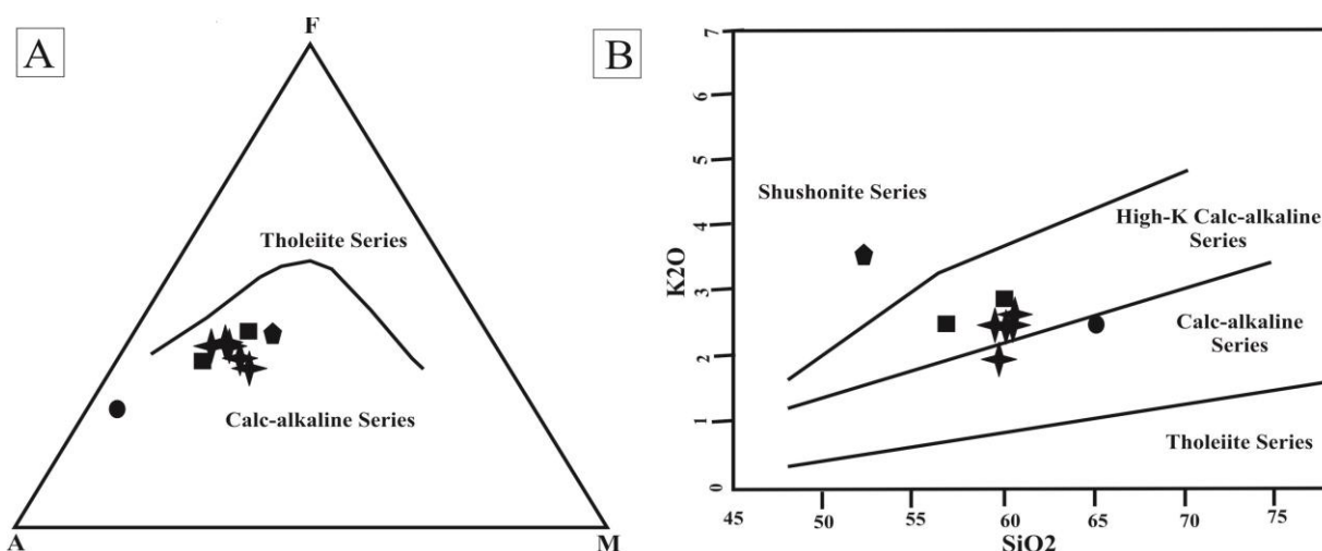
شکل ۹- جایگاه سنگ‌های آتشفشانی خاور خوسف در: (A) نمودار AFM (Irvine and Baragar, 1971); (B) نمودار K_2O در برابر SiO_2 (Peccerillo and Taylor, 1976)
