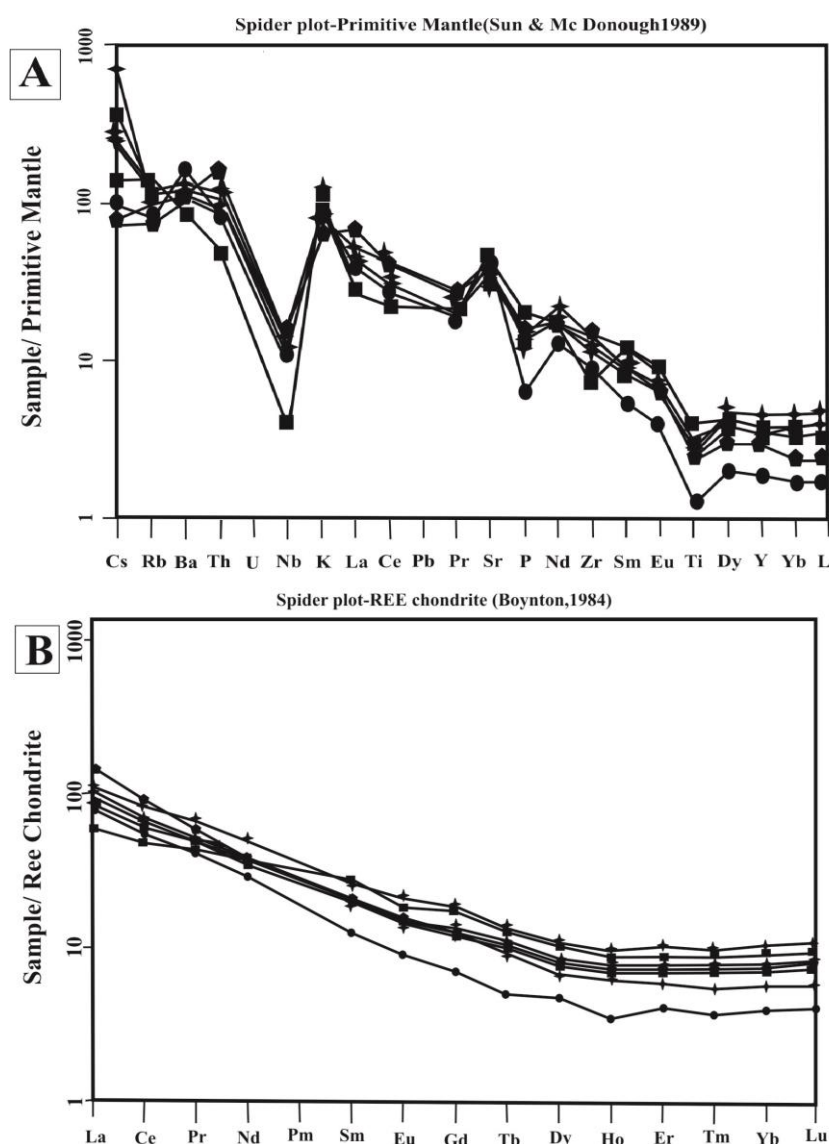
شکل ۱۰- سنگ‌های آتشفشانی و نیمه‌عمیق خاور خوسف در نمودار عنصرهای کمیاب بهنجار شده در برابر: (A) ترکیب گوشته اولیه (Sun and McDonough, 1989)؛ (B) ترکیب کندریت (Boynton, 1984)
