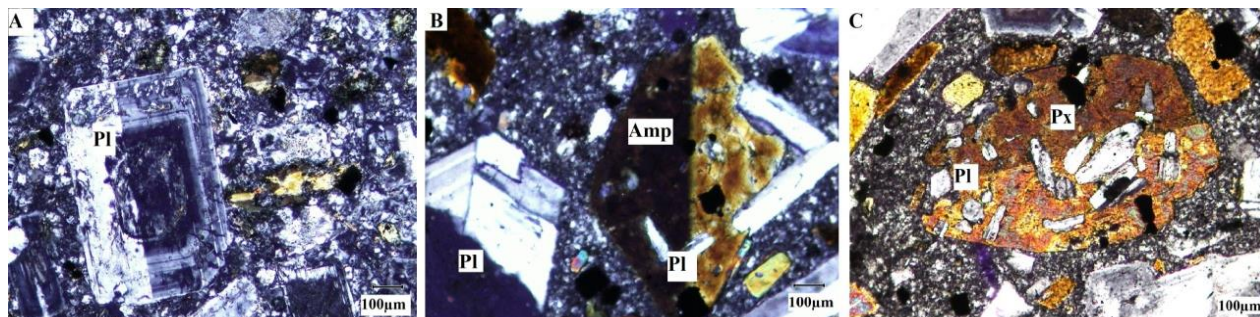
شکل ۳- آندزیت‌های خاور خوسف (جنوب‌باختری بیرجند): (A) درشت‌بلور پلاژیوکلاز با منطقه‌بندی نوسانی، ماکل کارلسباد و بافت غربالی؛ (B) ماکل ساده و بافت پویی کیلیتیک در آمفیبول؛ (C) ماکل ساده و بافت پویی کیلیتیک (پلاژیوکلاز درون پیروکسن) در پیروکسن (نور در همه تصاویرها XPL است)
